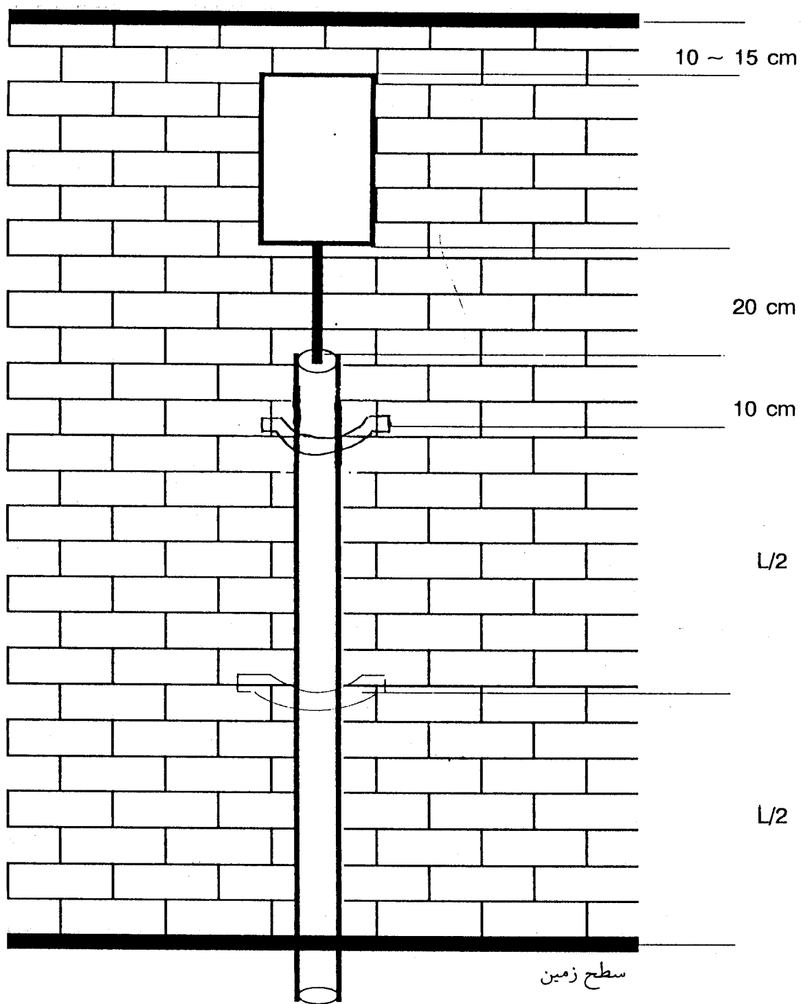
شکل نصب پست در ارتفاع ۱/۸ تا ۲/۵ متر
